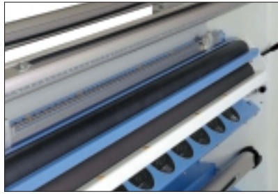
Ausgabeschneiderrollen zum Zuschneiden der Erzeugnisse während der Verarbeitung. Kühlventilatoren für lange Lauf- und Betriebszeiten.
