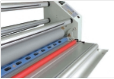
Zufahrtstisch mit Spannwellen und herunterklappbarer Druckführungsvorrichtung für eine gleichmäßige und optimale Materialbeschickung.
